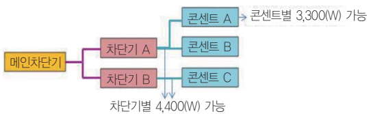
[그림] 가정 내 일반적인 전기배선(220V)의 예
