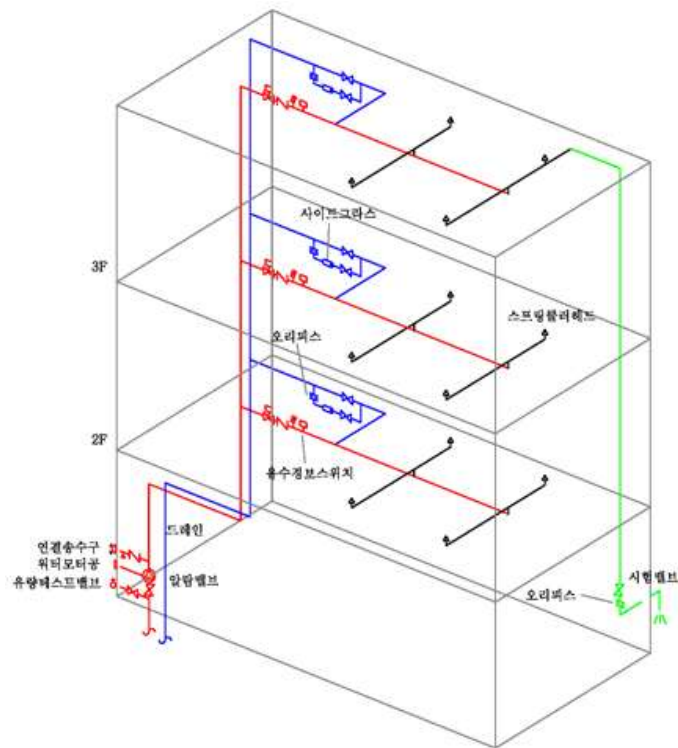
[그림 7-1] 습식설비의 시험밸브 위치
