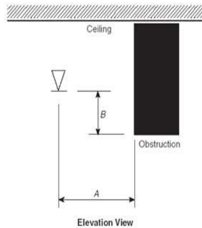
[그림 4-3] 살수장애를 피하기 위한 스프링클러헤드의 배치
