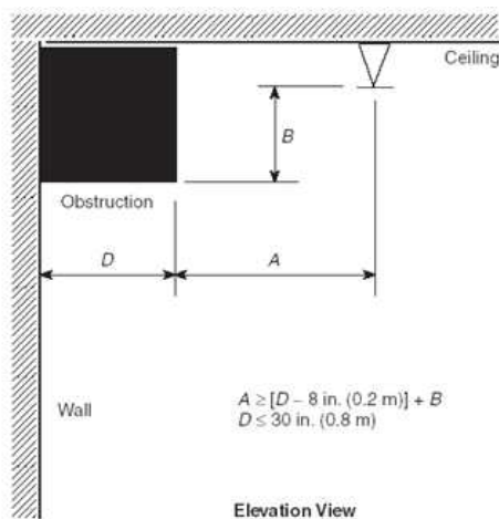
[그림 4-3] 살수장애를 피하기 위한 스프링클러헤드의 배치
