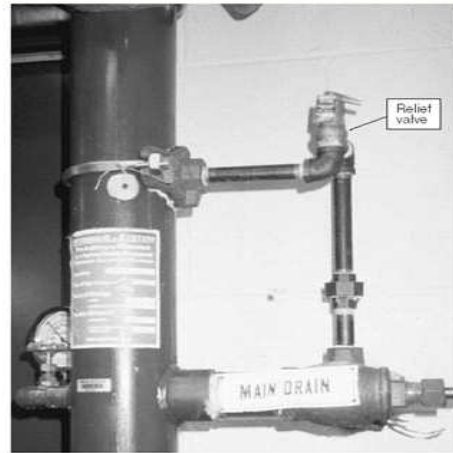
[그림 2-5] 격자형설비의 릴리프밸브
