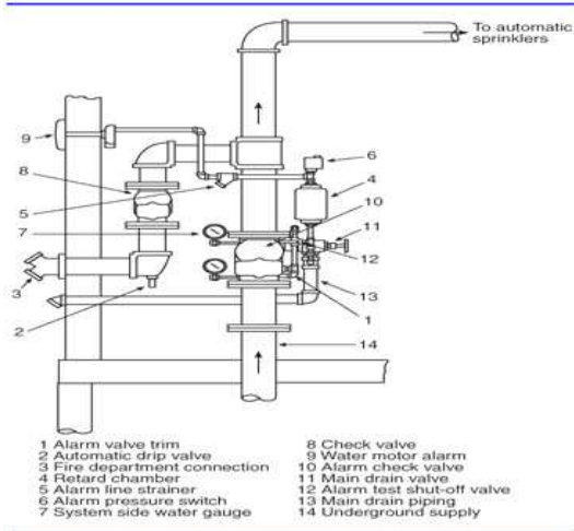
[그림 2-4] 습식밸브 입면도
