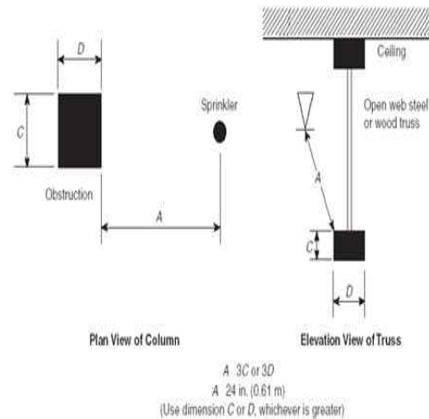
[그림 4-3] 살수장애를 피하기 위한 스프링클러헤드의 배치
