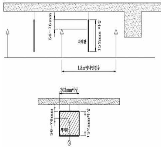
[그림 4-2] 스프링클러헤드 간 최소간격
